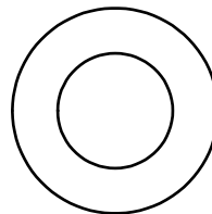
(C7) 1/2"(I.D.) FLAT WASHER Ø25X2T QTY.2
