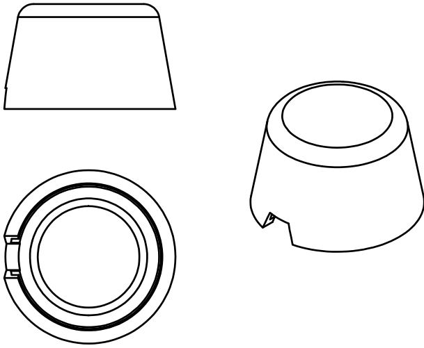
(C8)1/2" BOLT CAP(9212-024) QTY.4
