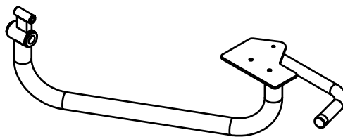
O[1PCS] 8220-162 Ø20X260L
